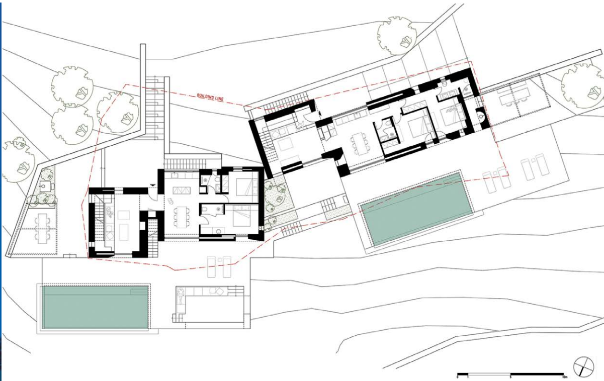
ΚΑΤΟΨΗ ΙΣΟΓΕΙΟΥ GROUND FLOOR PLAN
